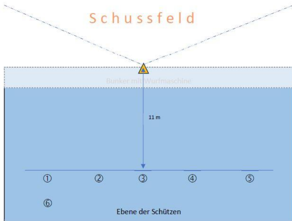
Schematischer Aufbau des Schießens zum TSN-Einzelmodul „Flinte bewegliches Ziel“ auf einer Ein-Maschinen-Anlage (jagdliches Trap-Schießen)
